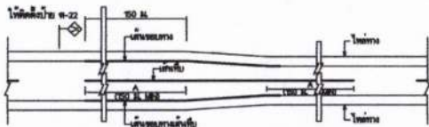
การตีเส้นจราจร กรณีความกว้างของจราจรลดลง SCALE A4 NTS.
