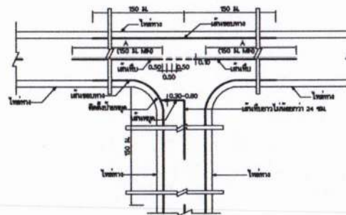
การตีเส้นจราจรทางแยก SCALE A4 NTS.
