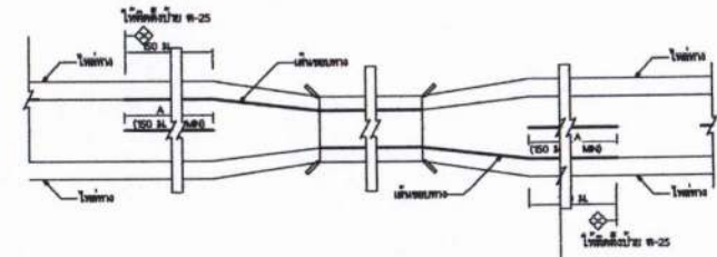
การตีเส้นจราจรบริเวณสะพาน SCALE A4 NTS.
