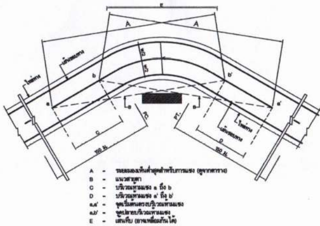
การตีเส้นจราจรบริเวณโค้งวง SCALE A4 NTS.
