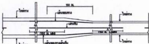
การตีเส้นจราจร กรณีความกว้างไหล่ทางลดลง SCALE A4 NTS.
