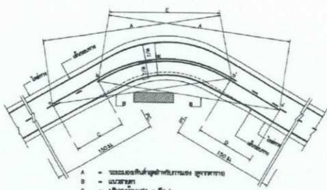
กรณีเส้นจราจรกับบริเวณยกพื้นสูง
