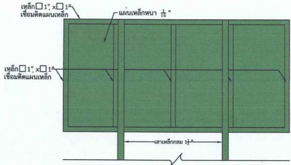
รายละเอียดป้ายโครงการ SCALE A4 / 125
