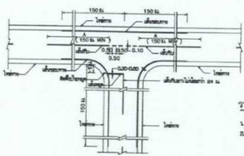
กรณีเส้นจราจรกับขอบทาง
