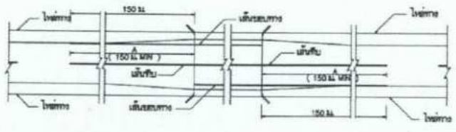
กรณีความกว้างของทางวิ่งที่ความกว้างผิวจราจร
