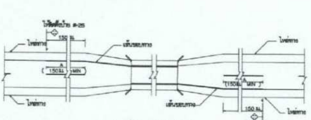
กรณีเส้นจราจรกับบริเวณยกพื้นสูง
