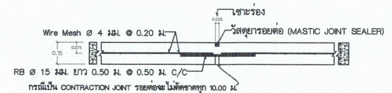
ขยายรอยต่อ EXPANSION JOINT SCALE A4 / 1:25
