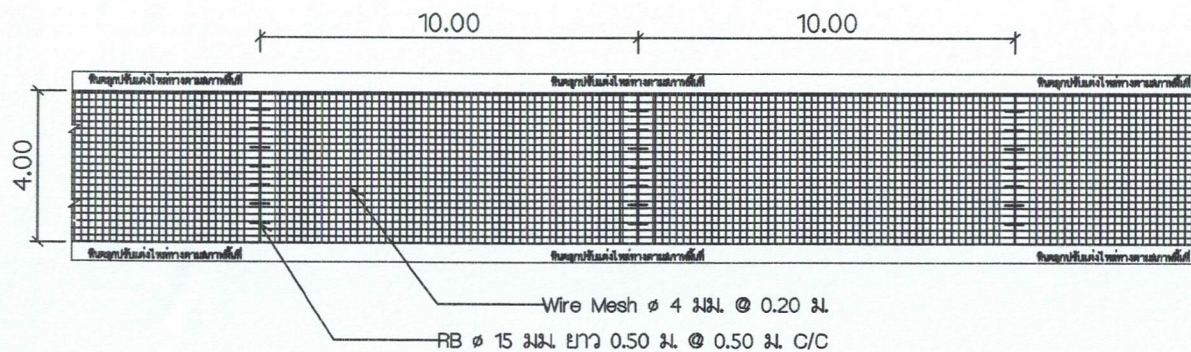
แปลนแสดงการเสริมเหล็กและรอยต่อ SCALE A4 / 1:200
