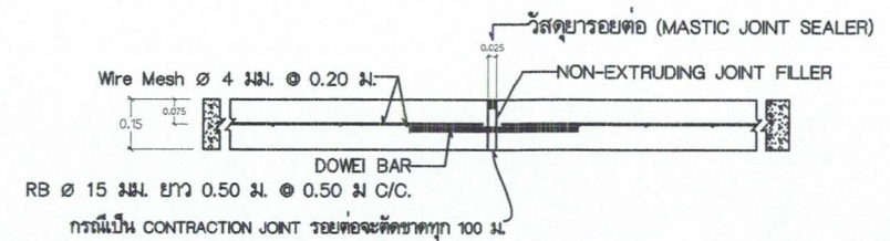
ขยายรอยต่อ EXPANSION JOINT SCALE A4 / 1:25
